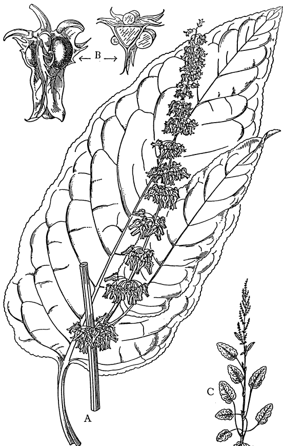
Rumex obtusifolius
