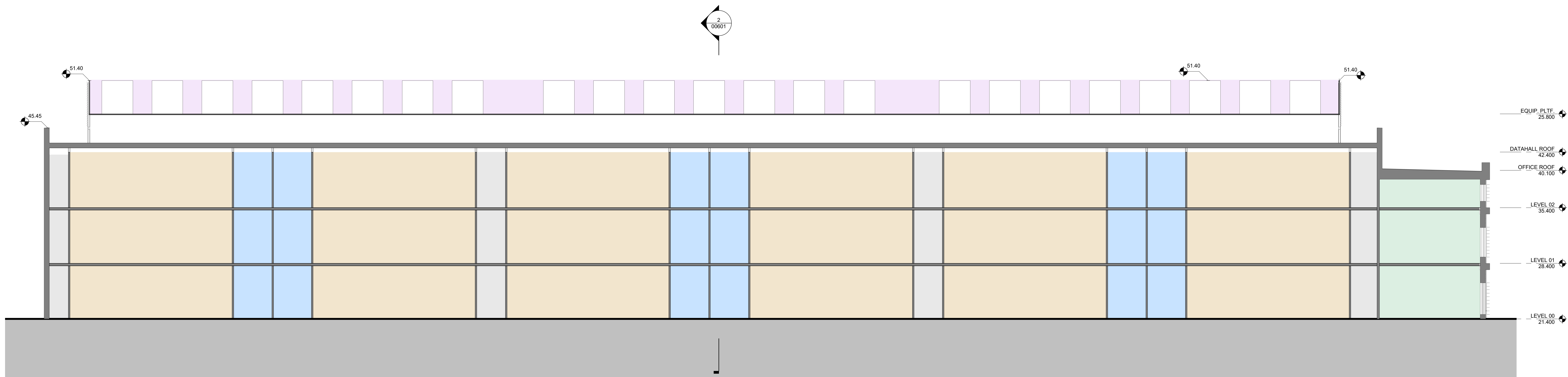
1 SECTION E/W 1 : 200
